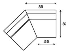
FC 111 hoekelement 45°
